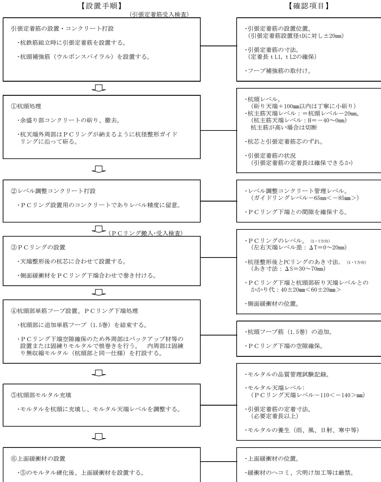
図4.1.5 PCリング及び引張定着筋の設置手順フロー（先付け方式）
