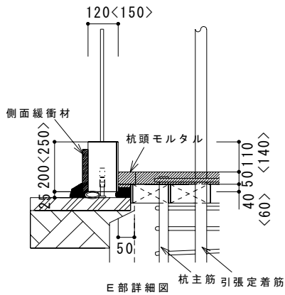
図 4.1.6(3) P C リング及び引張定着筋の設置手順(手順⑤～⑥)
