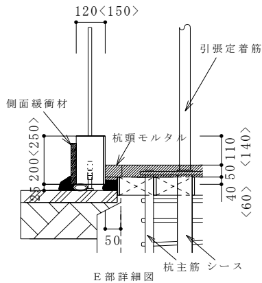
図 4.1.4(3) PCリング及び引張定着筋の設置手順(手順⑤～⑥)
