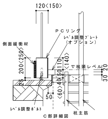
図 4.1.6(2) PCリング及び引張定着筋の設置手順(手順③～④)
