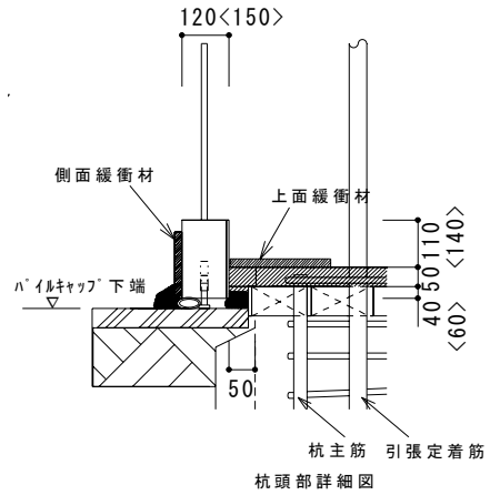
杭頭部詳細図
