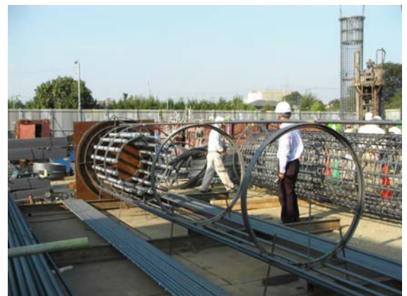
写真 2. 主筋取付け
