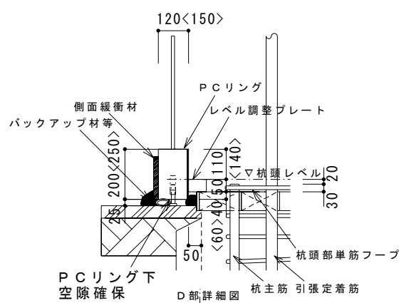
図 4.1.6(2) PCリング及び引張定着筋の設置手順(手順③～④)
