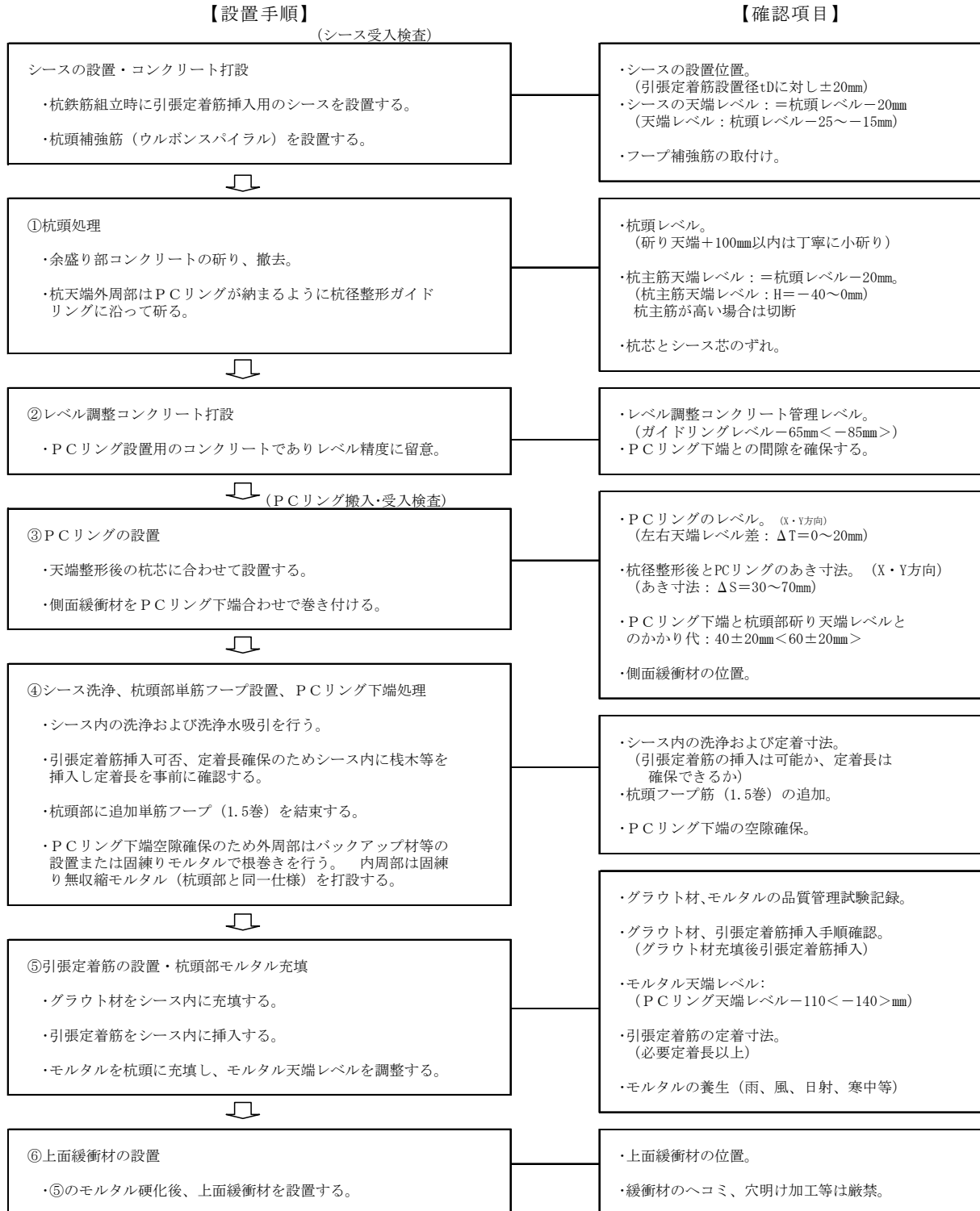
図4.1.3 PCリング及び引張定着筋の設置手順フロー(シース方式)
